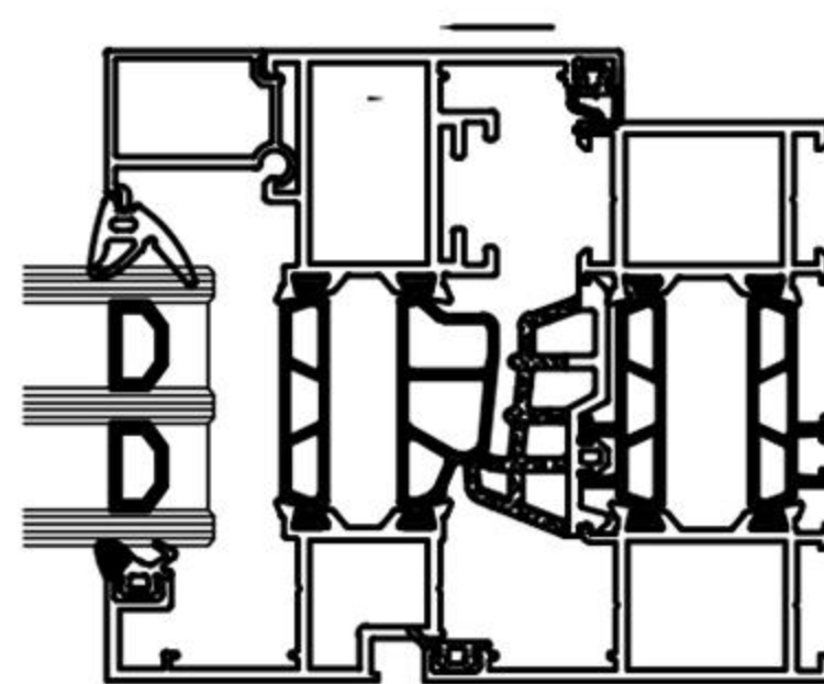
边框-开扇结构
