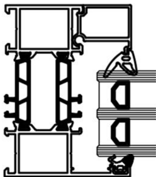
边框结构
