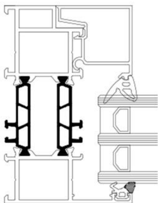
边框结构
